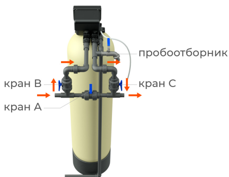
Подключение к водопроводу
