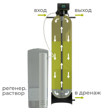
3. Прямая промывка
