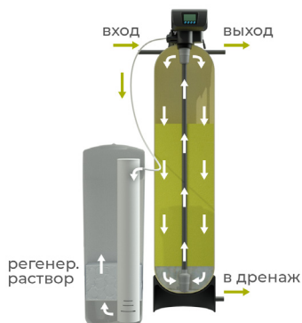
4. Заполнение водой реагентного бака
