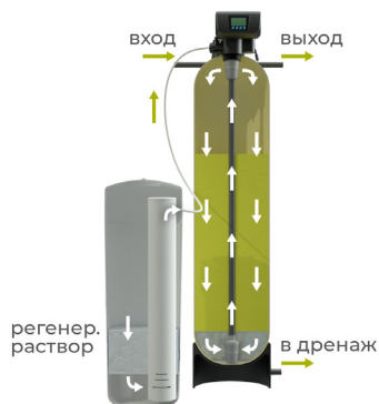
2. Поддача реагента
